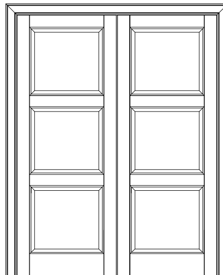
Каменя ДГ 8-8 двухстворчатая
