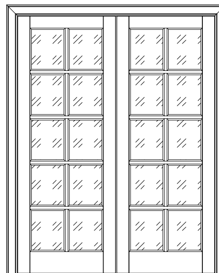
Кантри ДО-3 8-8 двухстворчатая
